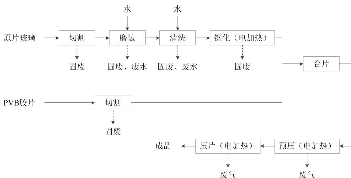
图 2-4 夹胶玻璃生产工艺流程和产污流程图（噪声伴随整个生产流程）
