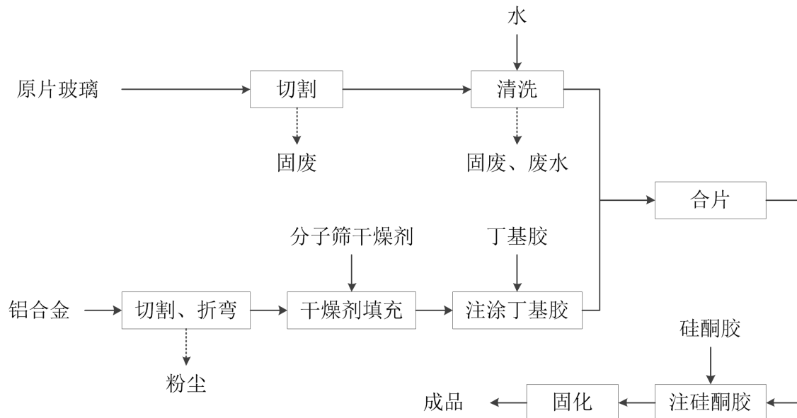
图 2-3 中空玻璃生产工艺流程和产污流程图（噪声伴随整个生产流程）
