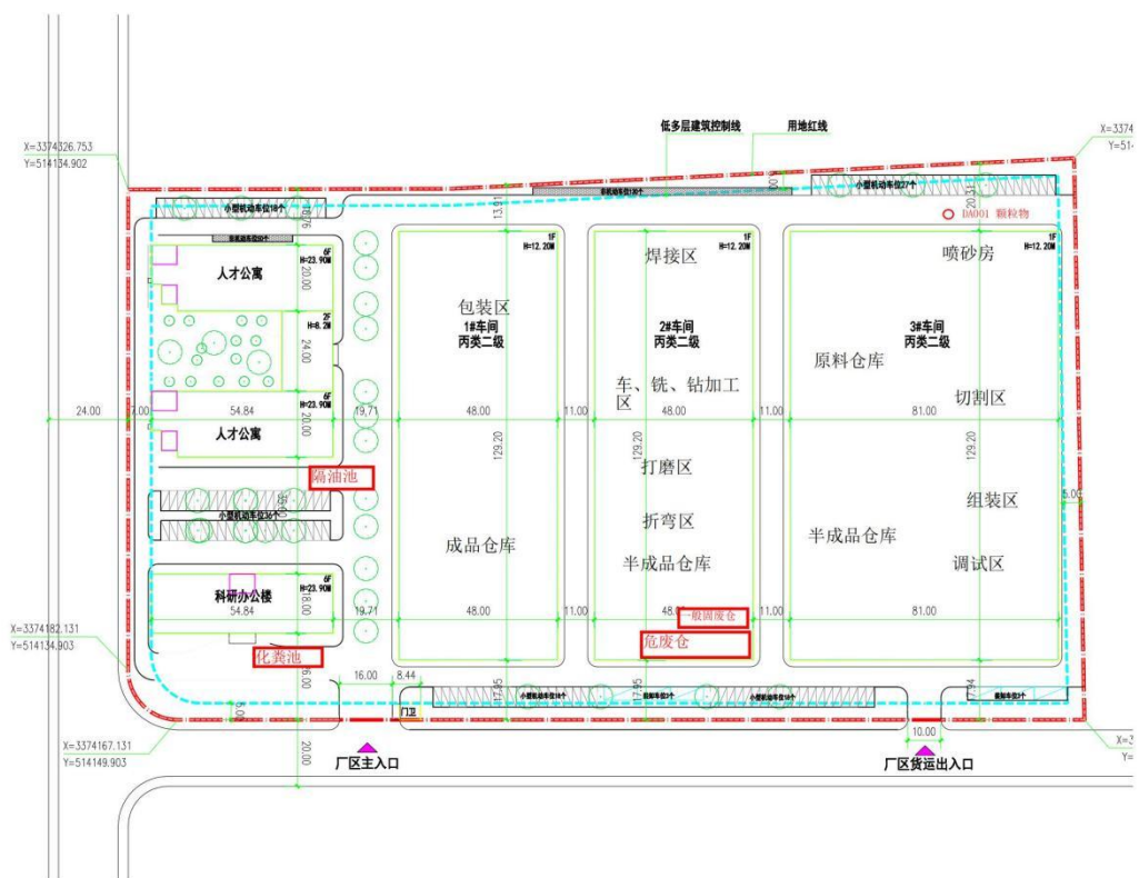
图 2-1 厂区平面布置图
